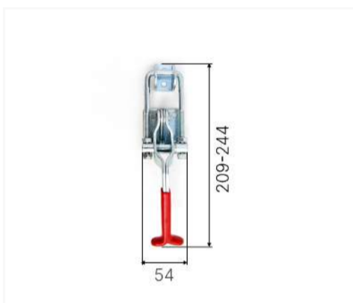
Замок В-240 (нержавеющая сталь)
