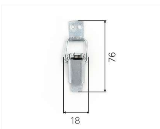
Замок Р-26 (живчик с пружиной)
