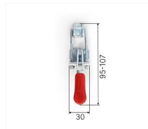
Замок В-110 (нержавеющая сталь)
