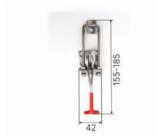
Замок В-180 (нержавеющая сталь)
