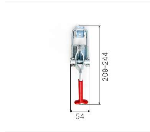
Замок В-240 (нержавеющая сталь)
