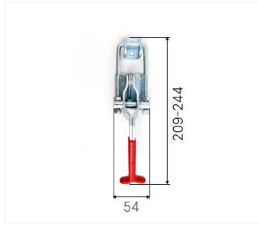
Замок В-240 (цинк)
